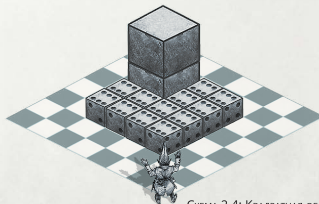
СХЕМА 2.4: КВАДРАТНАЯ ОБЛАСТЬ С ПОЛНЫМ УКРЫТИЕМ
