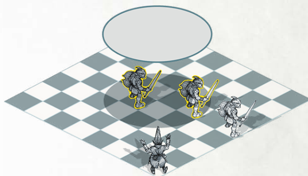
СХЕМА 2.2: ШАБЛОН КРУГА
