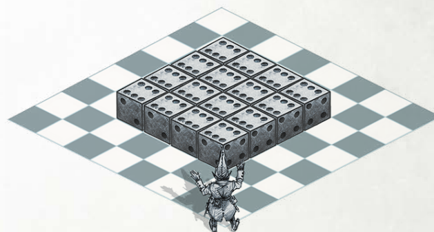
СХЕМА 2.3: КВАДРАТНАЯ ОБЛАСТЬ С ИСПОЛЬЗОВАНИЕМ ЖЕТОНОВ
